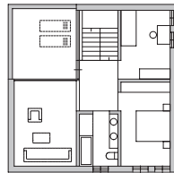
Variante OG mit Terrasse und Luftraum
