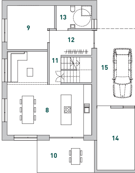
Erdgeschoss
